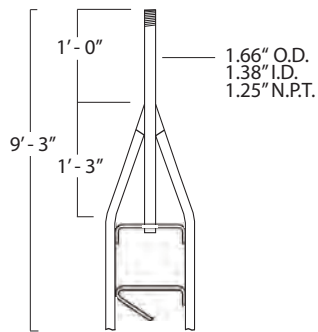
TOP SECTION 25AG1
